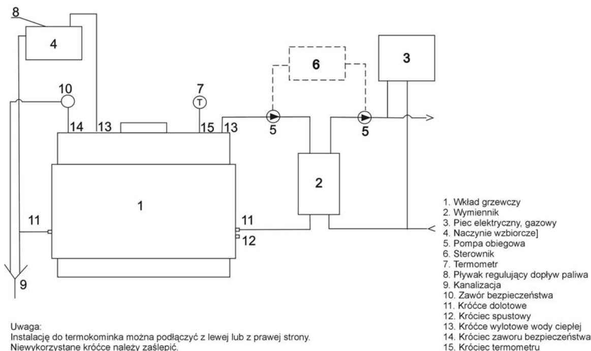
Przykładowy uproszczony projekt instalacji c.o.
